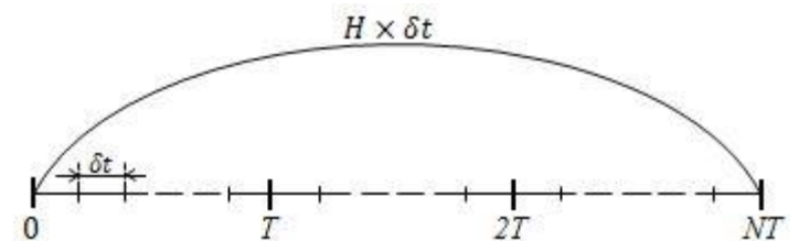
Fig. 1. L'horizon fini réparti en N intervalles périodiques ( N=1,2,\dots )
